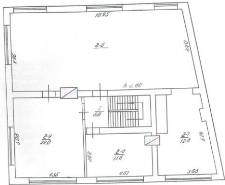
2 поверх
