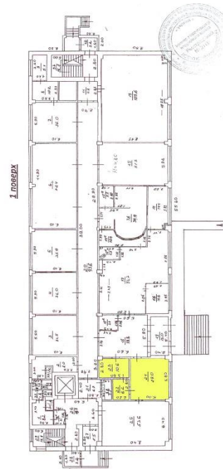
ПОВЕРХОВИЙ ПЛАН на нежитлову будівлю літер «А-4» вул. Старошишківська №5-а м. Харків
