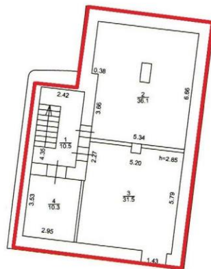
Підвал літ. "Б"
